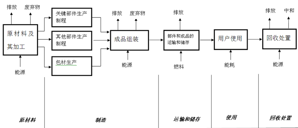
图 A.1 吸油烟机生命周期系统边界图
