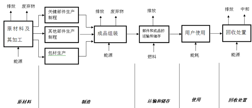
图 A.1 家用电冰箱生命周期系统边界图
