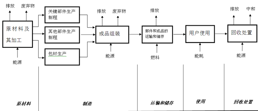
图A.1 商用电磁灶生命周期系统边界图
