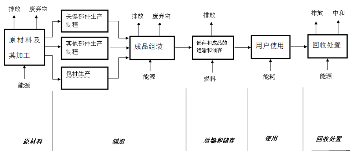
图 A.1 房间空气调节器生命周期系统边界图
