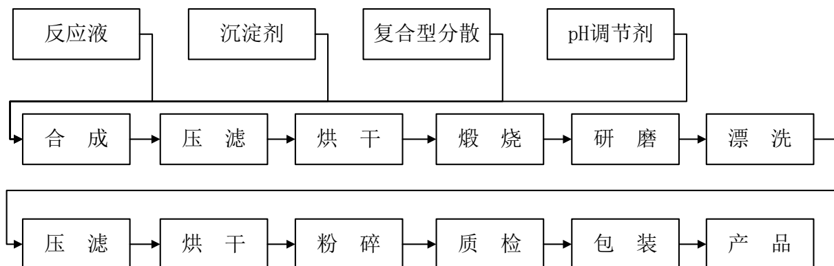
图 B.1 金属氧化物混相颜料产品生命周期系统边界图
