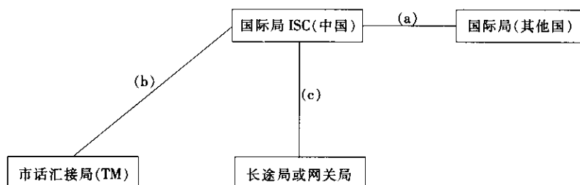
图1 国际去话呼叫的连接示意
