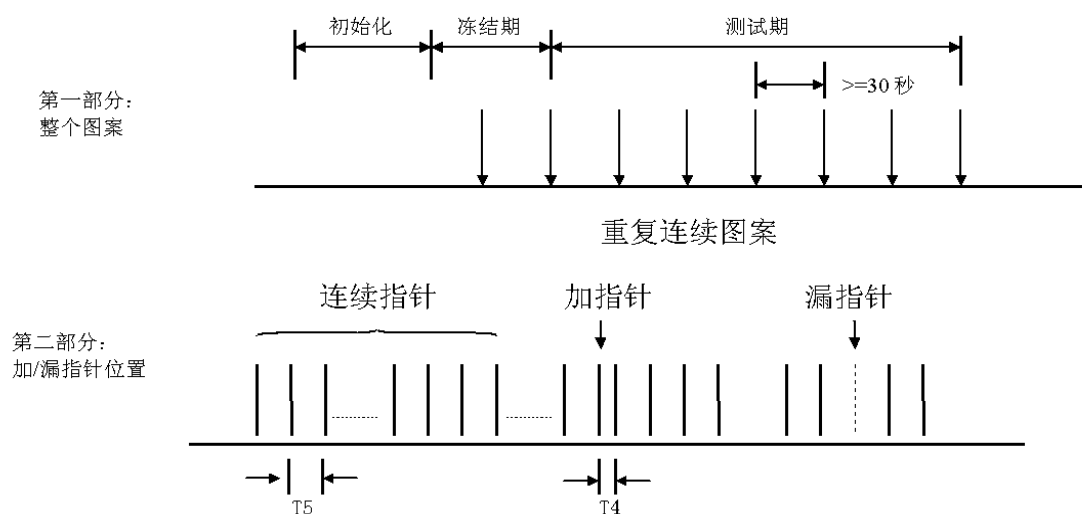
图 4.2.9 指针测试序列
