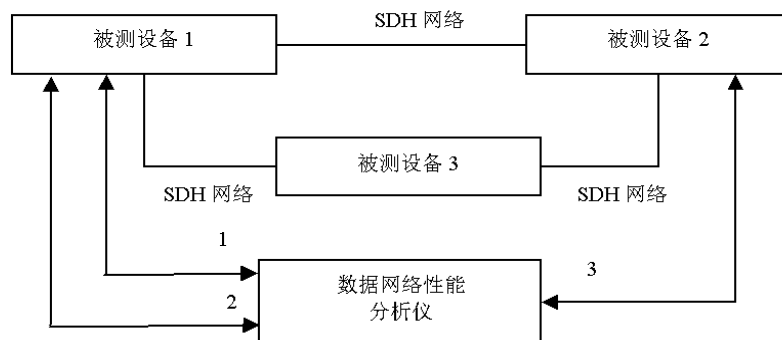
图 4.3.3-1 多端口到单端口的以太网业务汇聚测试连接示意图
