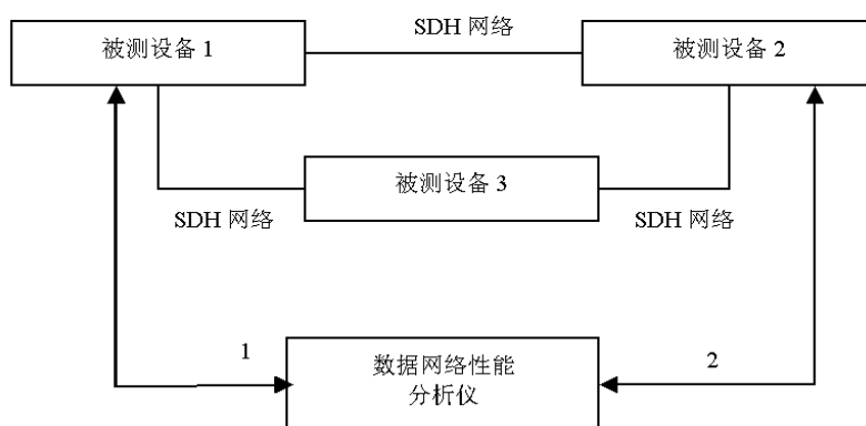
图 4.3.3-2 多分支网元到中心网元的以太网业务汇聚测试连接示意图
