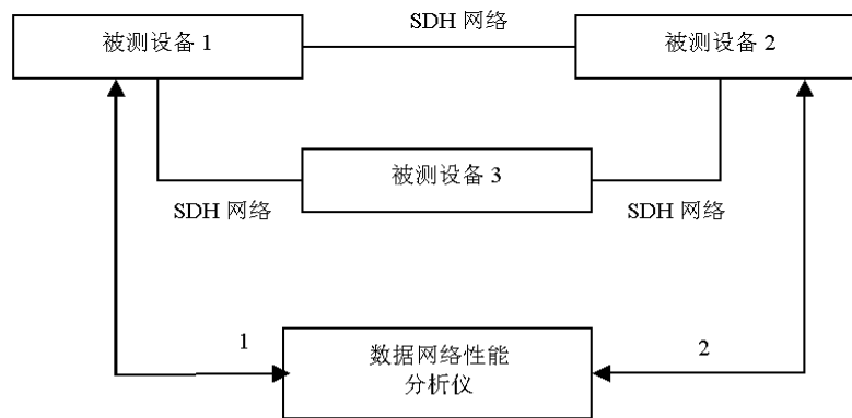
图 5.1.6 以太网业务保护（基于 SDH）测试连接图
