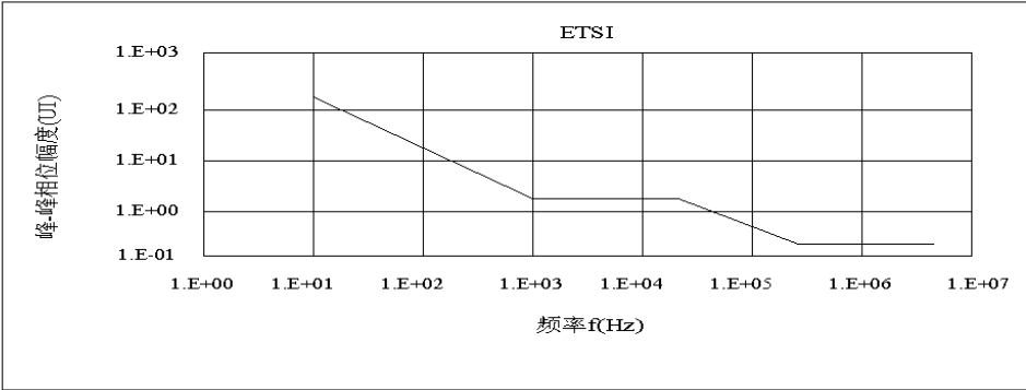
4. 2. 5-4 STM-4 光接口的输入抖动容限模板
