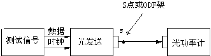
图 4.2.1 平均发送光功率测试连接示意图
