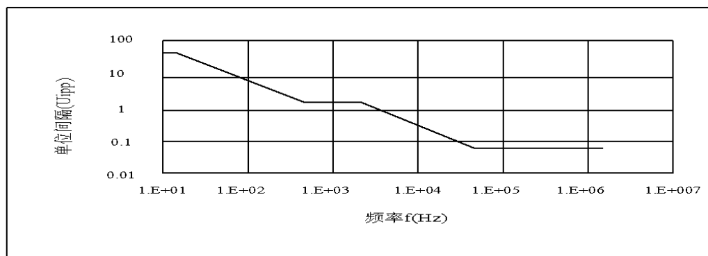
图 4.2.5-2 STM-1 电接口的输入抖动容限模板
