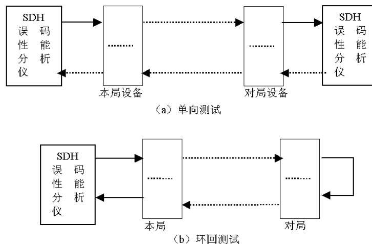
图 5.1.1 系统误码性能测试连接示意图
