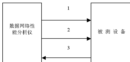
图 4.3.2-2 VLAN 优先级测试示意图
