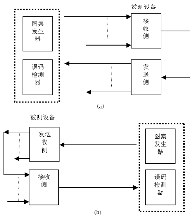
图 4.2.5-1 SDH 输入抖动容限/频偏测试连接示意
