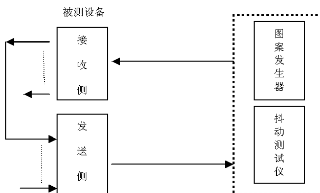
图 4.2.4 SDH 设备固有抖动测试连接示意图
