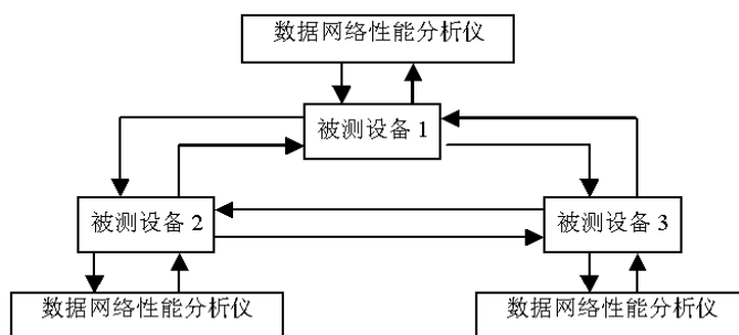
图 5.1.4 ATM 系统信元传送质量测试连接图
