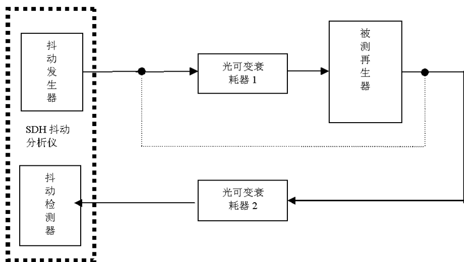
图 4.2.10-1 再生器抖动转移测试连接示意图
