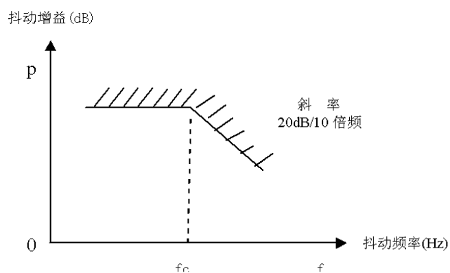
图 4.2.10-2 再生器抖动转移特性模板
