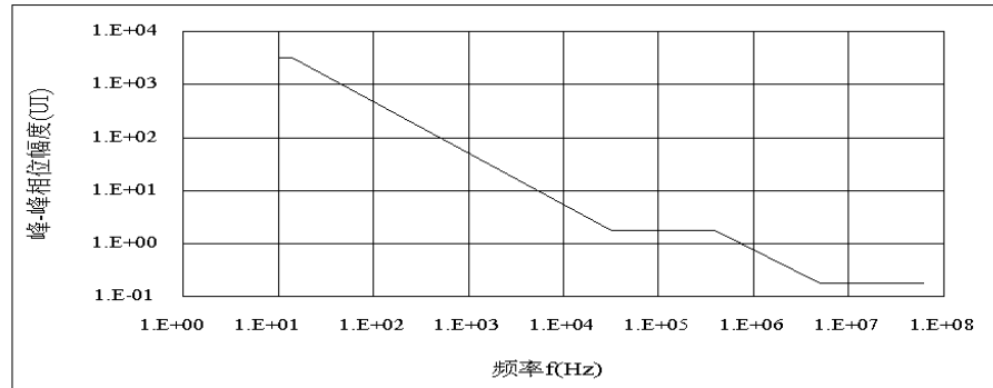
图 4.2.5-6 STM-64 光接口的输入抖动容限模板
