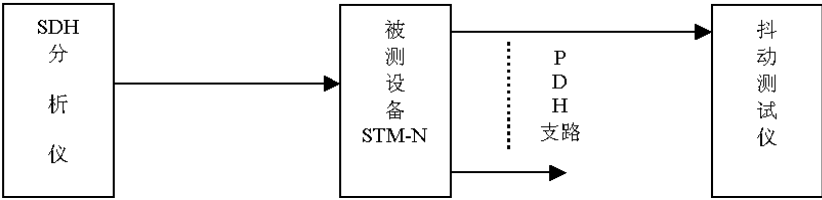
图 4.2.8 SDH 设备 PDH 接口的映射/结合抖动测试示意图
