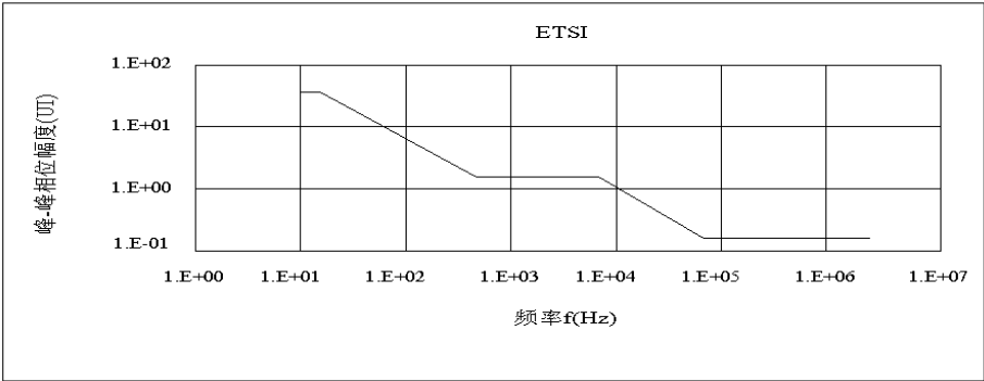
图 4. 2. 5-3 STM-1 光接口的输入抖动容限模板
