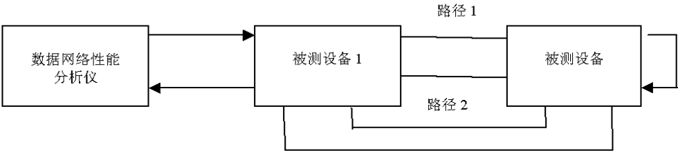
图 4. 3. 1-5 LCAS 功能测试示意图
