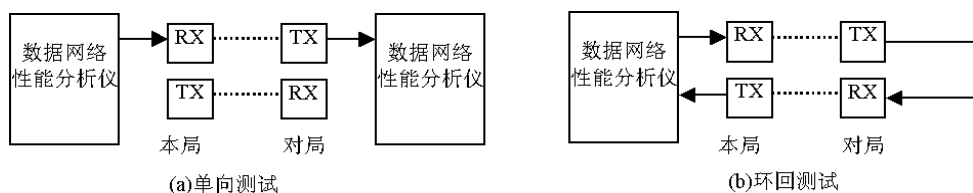
图 5.1.3 以太网系统性能测试连接示意图
