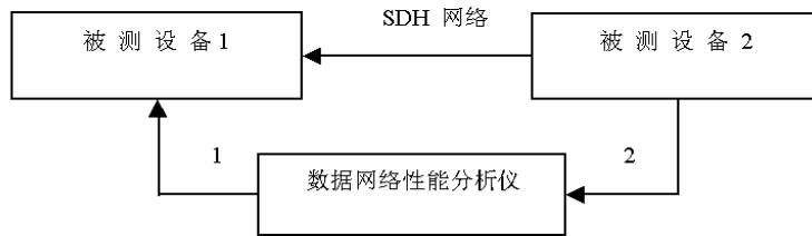
图 4.3.1-6 吞吐量/背靠背测试示意图
