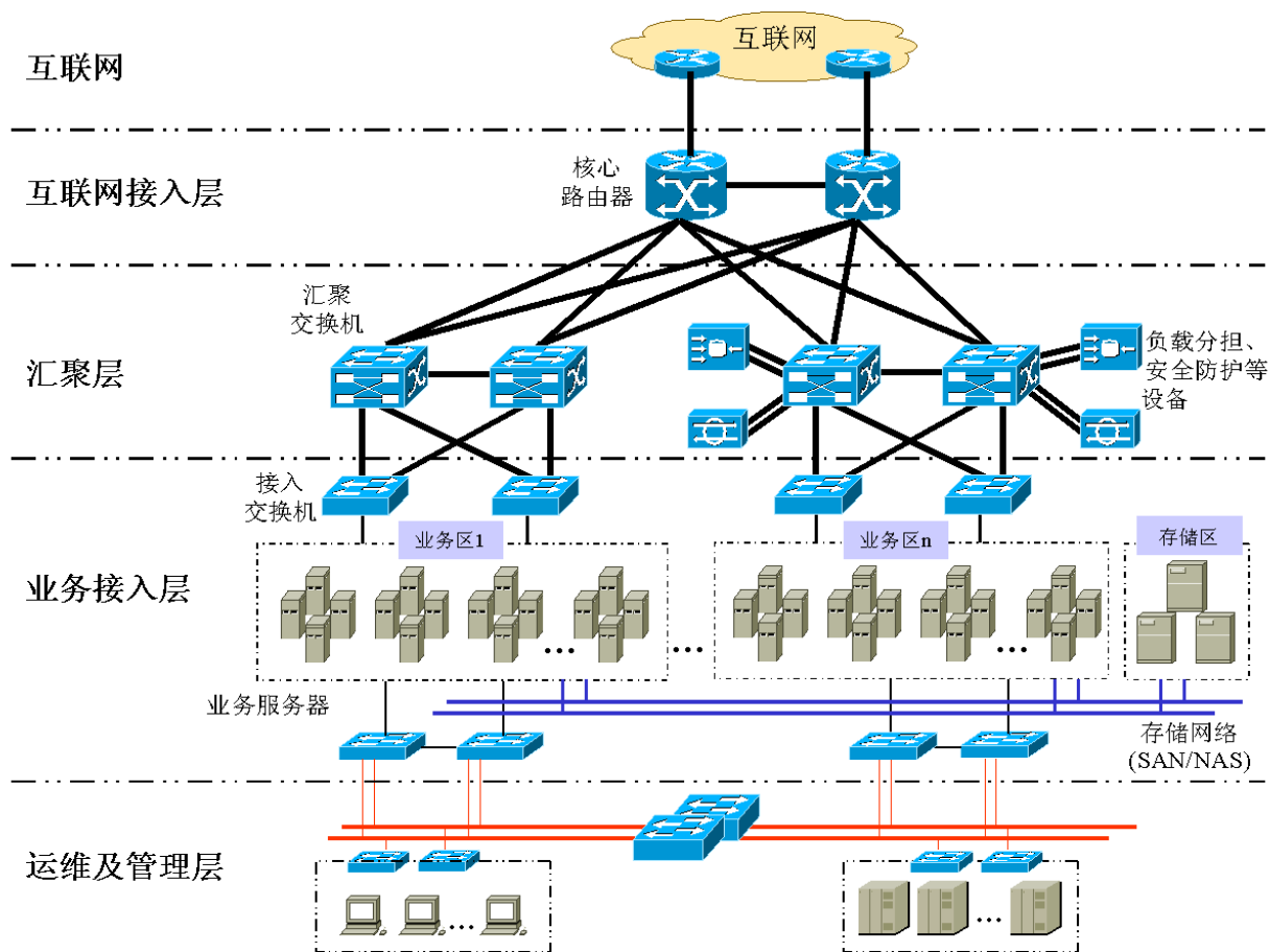
图 7.1.1 IDC 网络结构示意图
