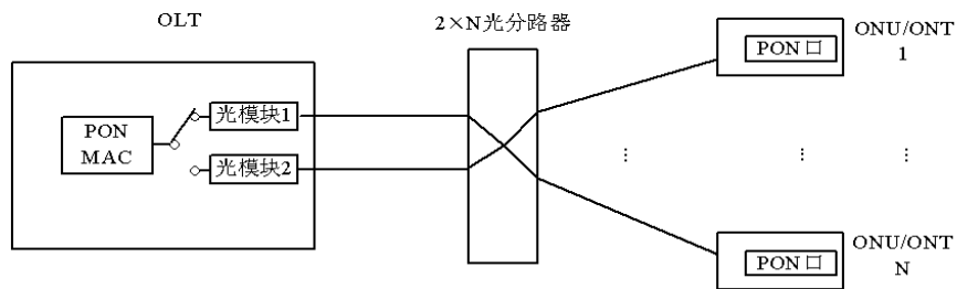
图4.6.1-1 主干光纤保护倒换类型a
