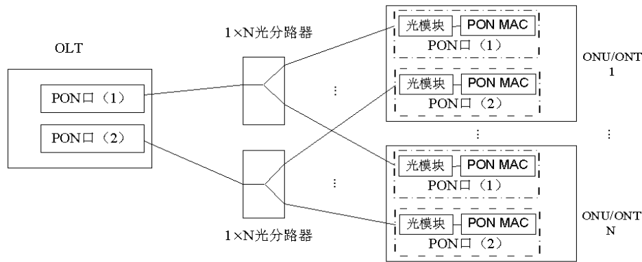
图4. 6. 1-4 全保护倒换类型d
