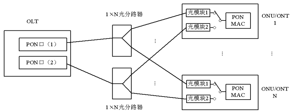
图4. 6. 1-3 全保护倒换类型c
