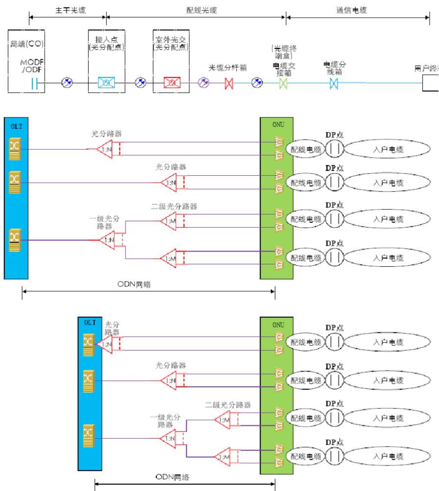
图 7.4.5 农村区域在 FTTCab 应用模式下 ODN 典型场景图
