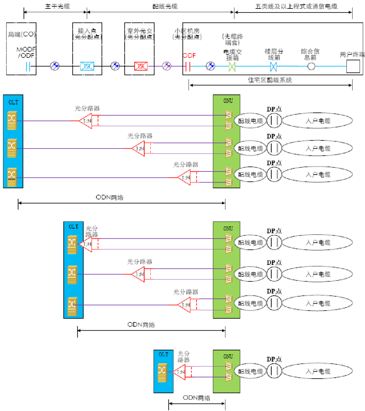
图 7.4.4-1 低层、多层和高层住宅在 FTTB 应用模式下 ODN 典型场景图
