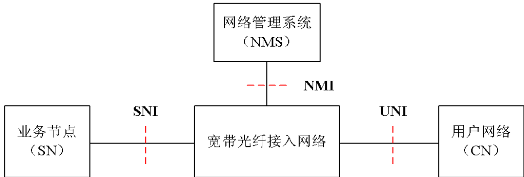
图 3.1.2 宽带光纤接入网的定界
