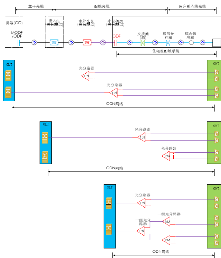
图 7.1.1 ODN 网络组成示意图(OLT 分别设置在局端、接入点和小区机房)
