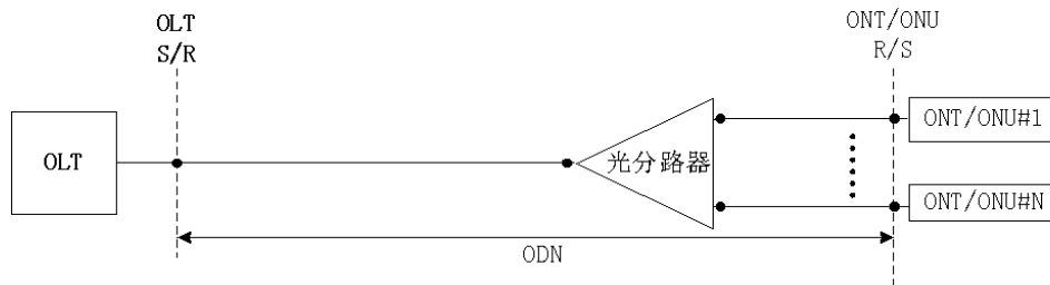
图 7.1.1 ODN 的定界
