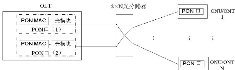
图4.6.1-2 主干光纤保护倒换类型b
