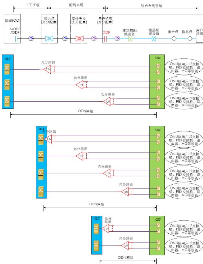
图 7.4.6-4 建筑群商务楼在 FTTC 应用模式下 ODN 典型场景图
