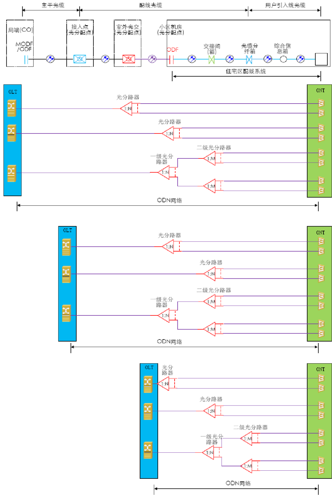
图 7.4.3 低层、多层和高层住宅在 FTTH 应用模式下 ODN 典型场景图
