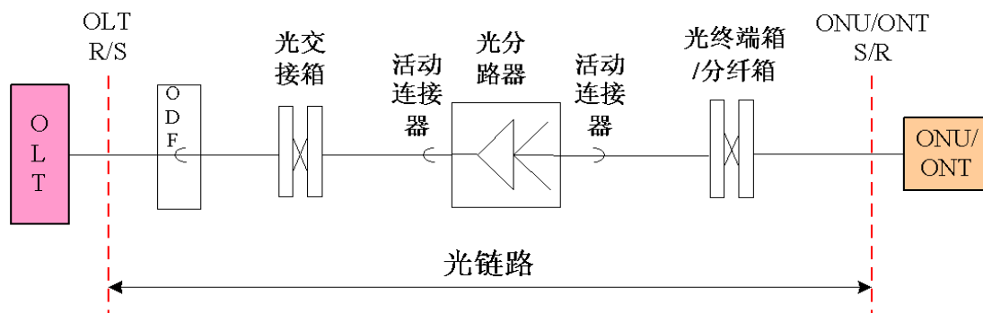
图8.2.1 ODN衰减指标设计的光链路参考模型
