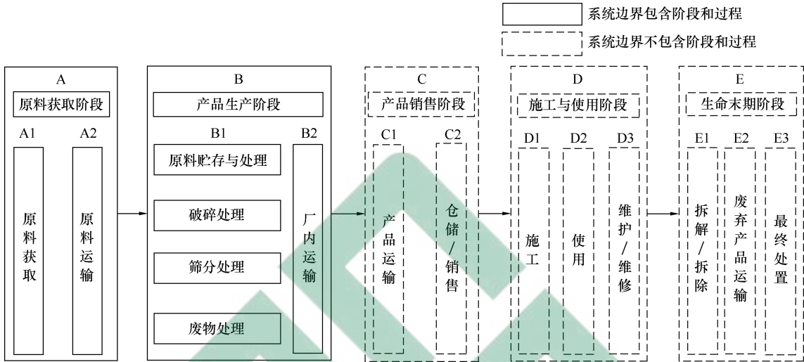
图 1 建设用砂、石产品碳足迹评价的系统边界图
