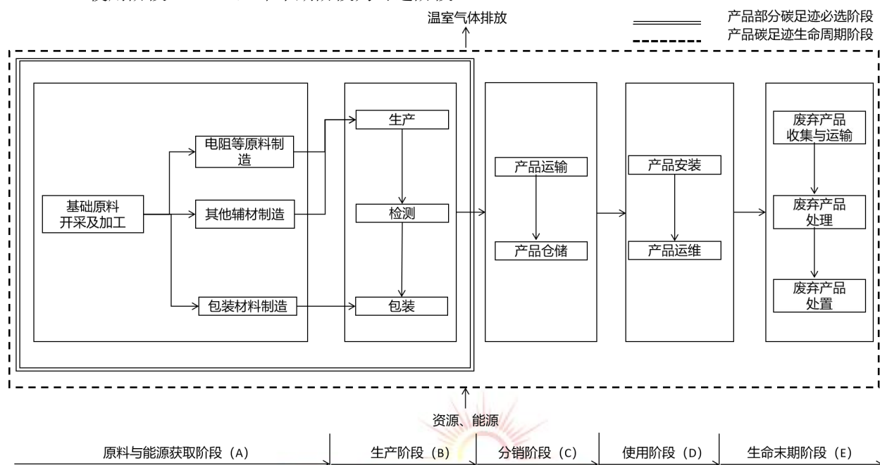
图1 光伏并网逆变器产品生命周期系统边界
