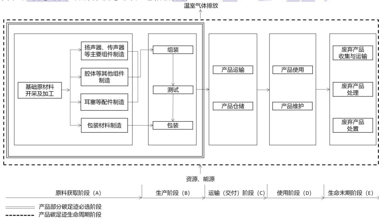
图 1 耳机产品碳足迹量化系统边界
