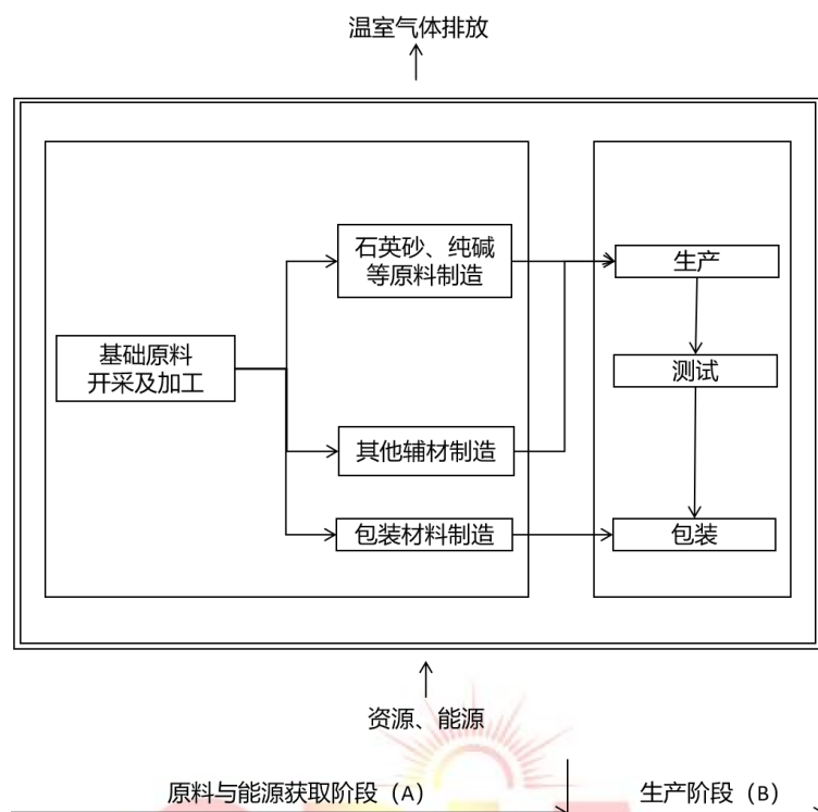
图1 光伏组件用玻璃产品生命周期系统边界
