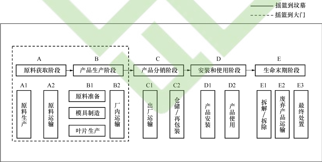
图1 风力发电机叶片产品碳足迹评价的系统边界图
