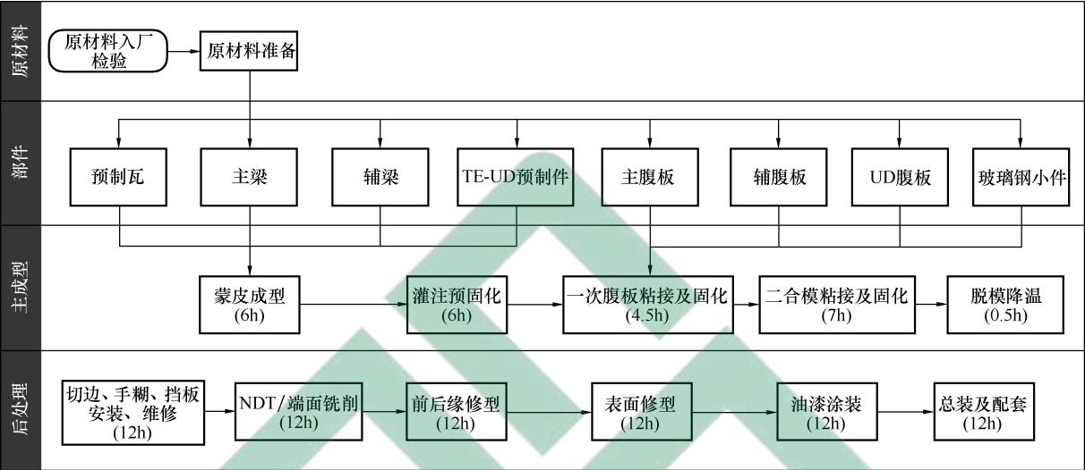
图 A.1 风电叶片生产典型工艺示例图
