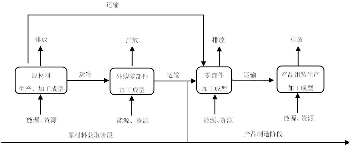
图1 电动机-压缩机产品碳足迹量化的系统边界示例
