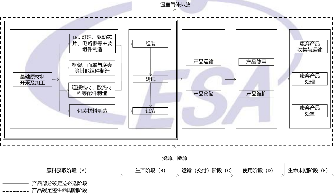
图 1 LED 显示屏产品碳足迹量化系统边界
