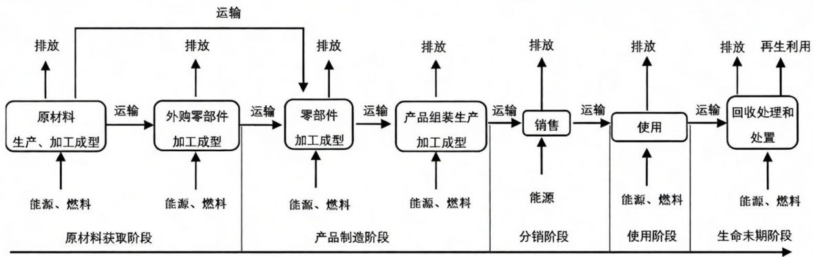
图1 室内加热器产品碳足迹量化的系统边界示例
