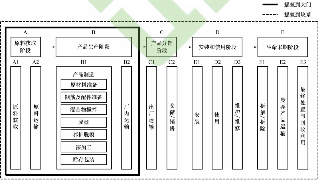
图1 水泥制品碳足迹评价的系统边界图
