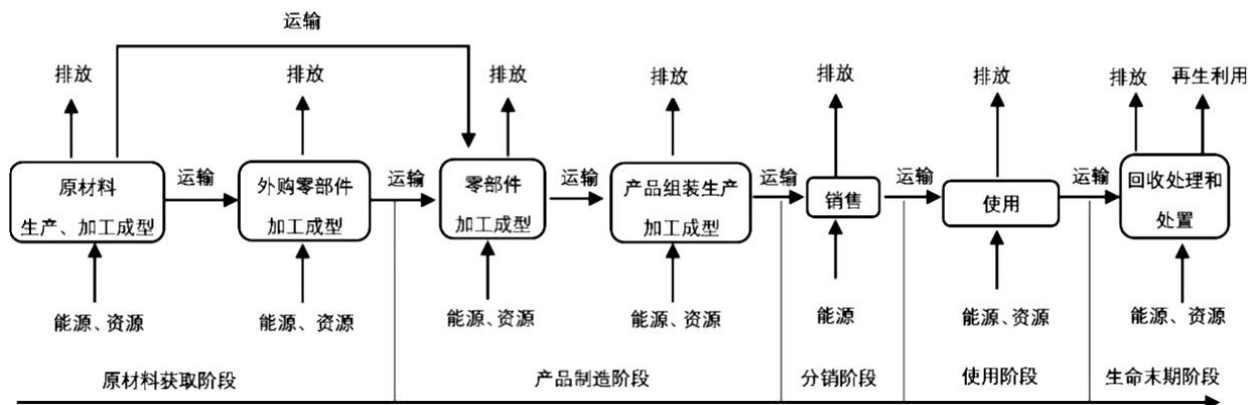
图1 储水式电热水器产品碳足迹量化的系统边界示例
