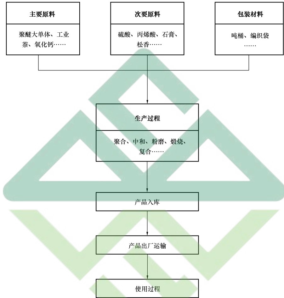
图 A. 1 混凝土外加剂产品生产工艺流程图
