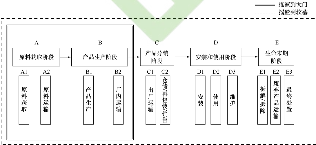
图 1 石材产品碳足迹评价的系统边界图
