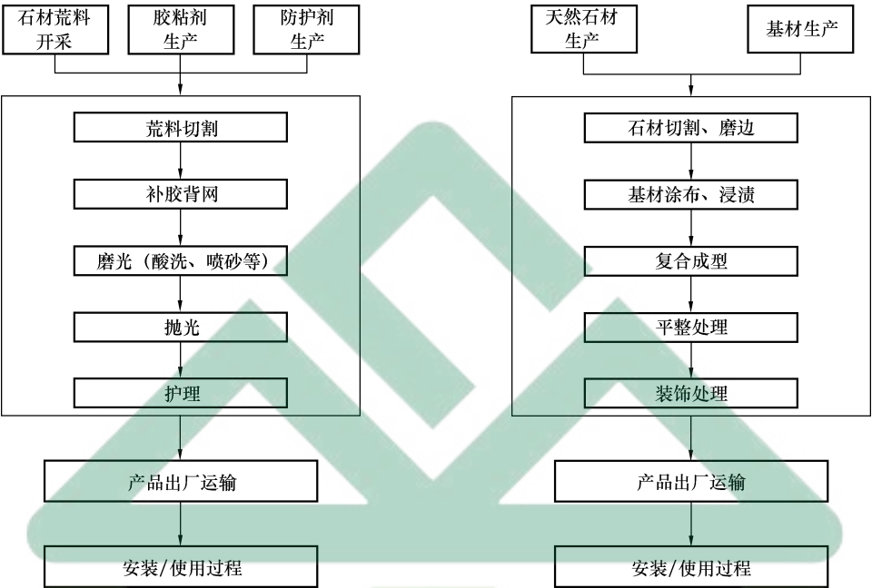
图 A.1 天然石材产品生产工艺流程图
