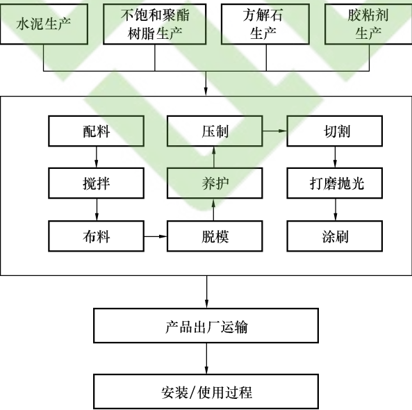
图 A.3 人造石材产品生产工艺流程图
