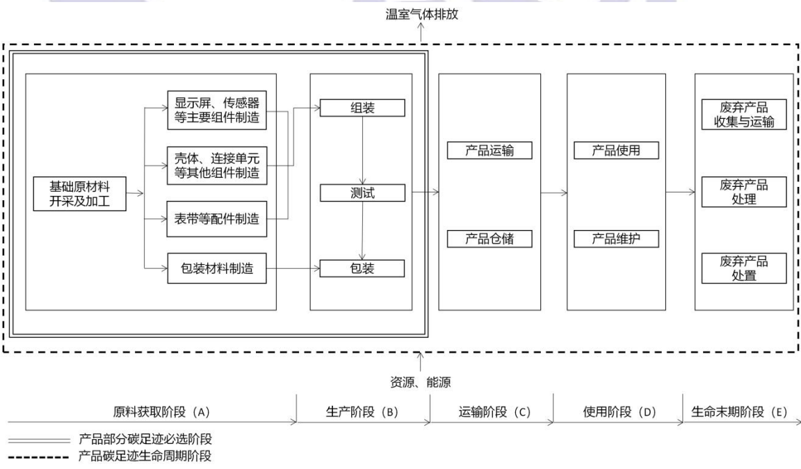
图 1 智能手表产品碳足迹量化系统边界
