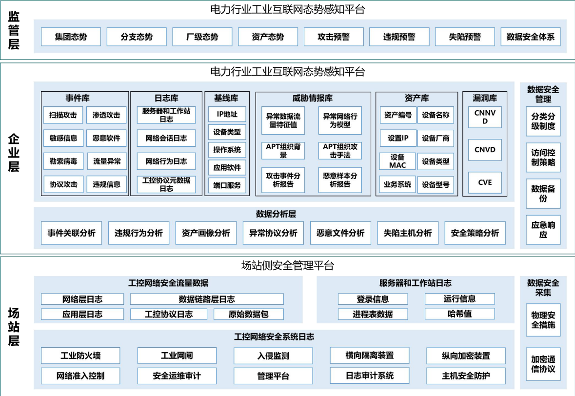
图 8-1 工业互联网安全与电力融合应用架构图
