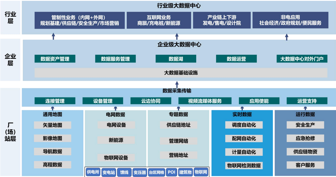
图 7-1 工业互联网数据与电力融合应用架构图
