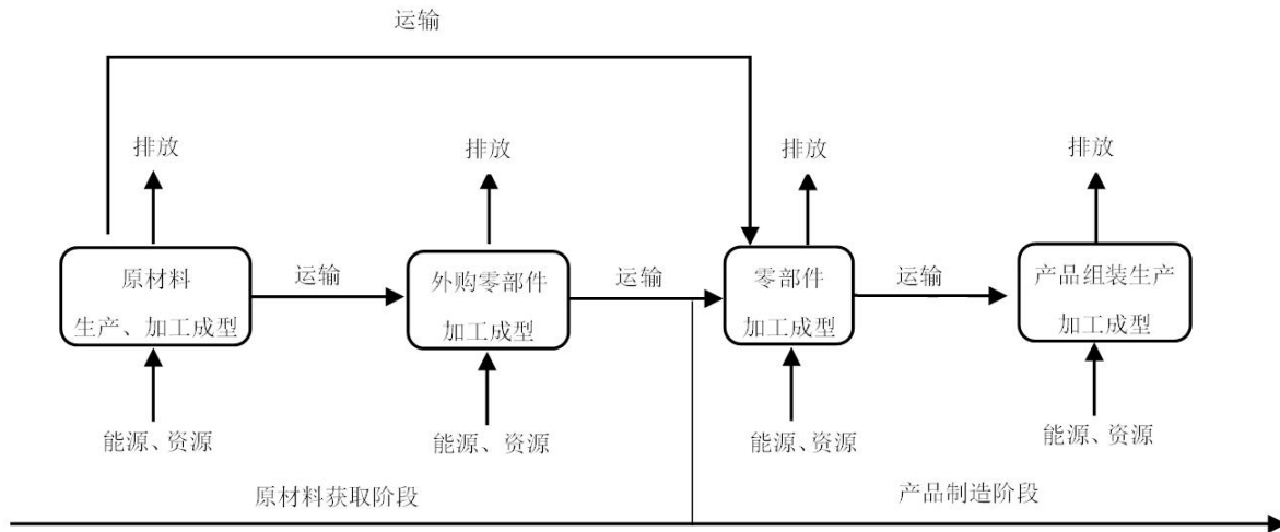
图1 小功率电动机产品碳足迹量化的系统边界示例
