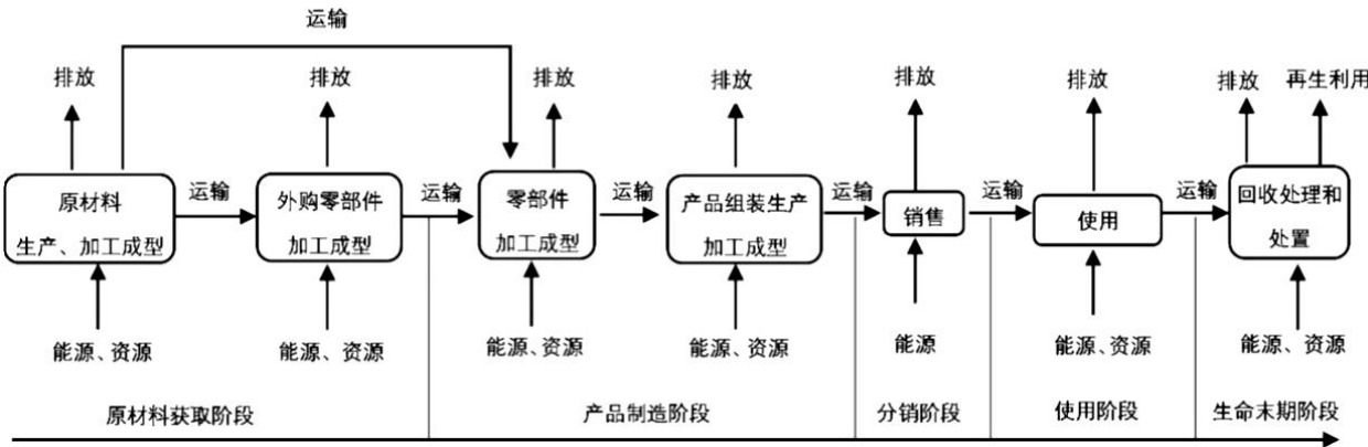
图1 空气净化器产品碳足迹量化的系统边界示例
