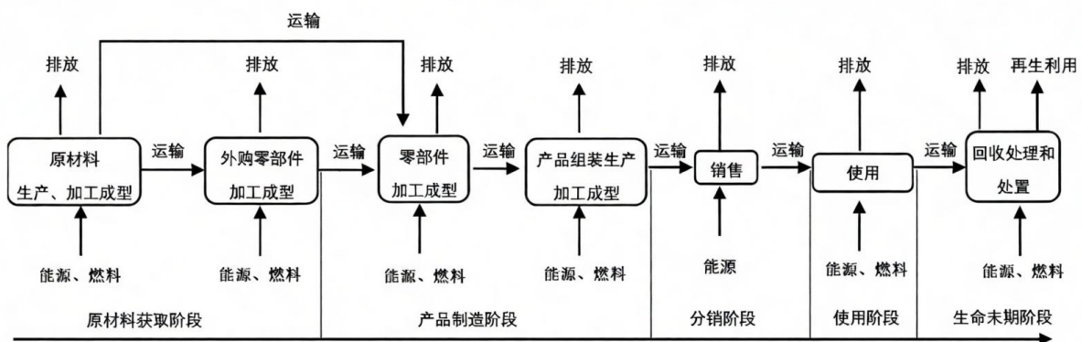
图1 电风扇产品碳足迹量化的系统边界示例
