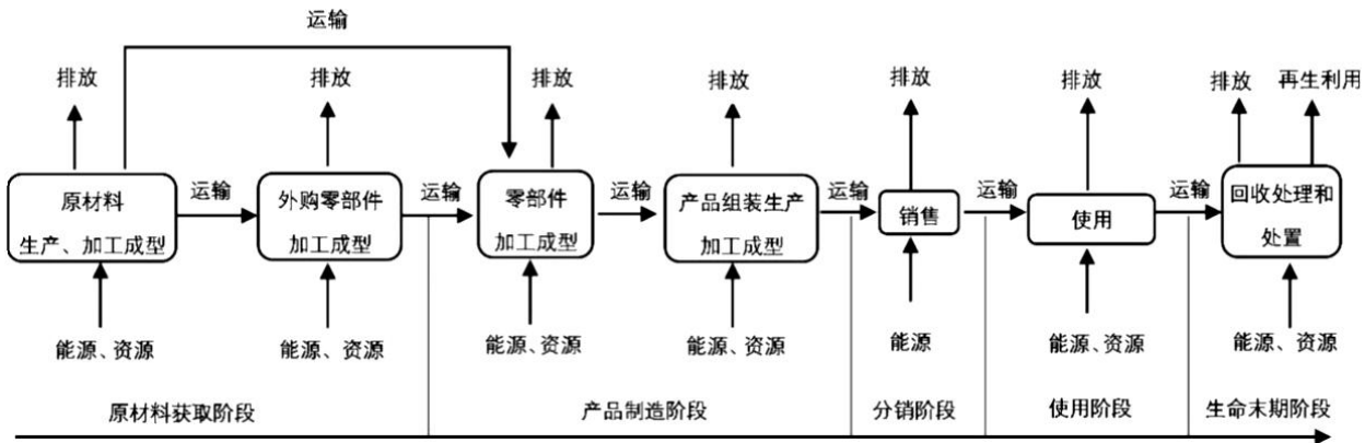
图1 电烤箱产品碳足迹量化的系统边界示例
