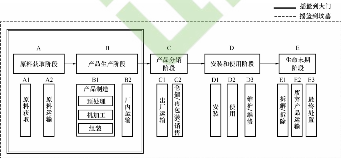
图 1 建筑门窗产品碳足迹评价的系统边界图
