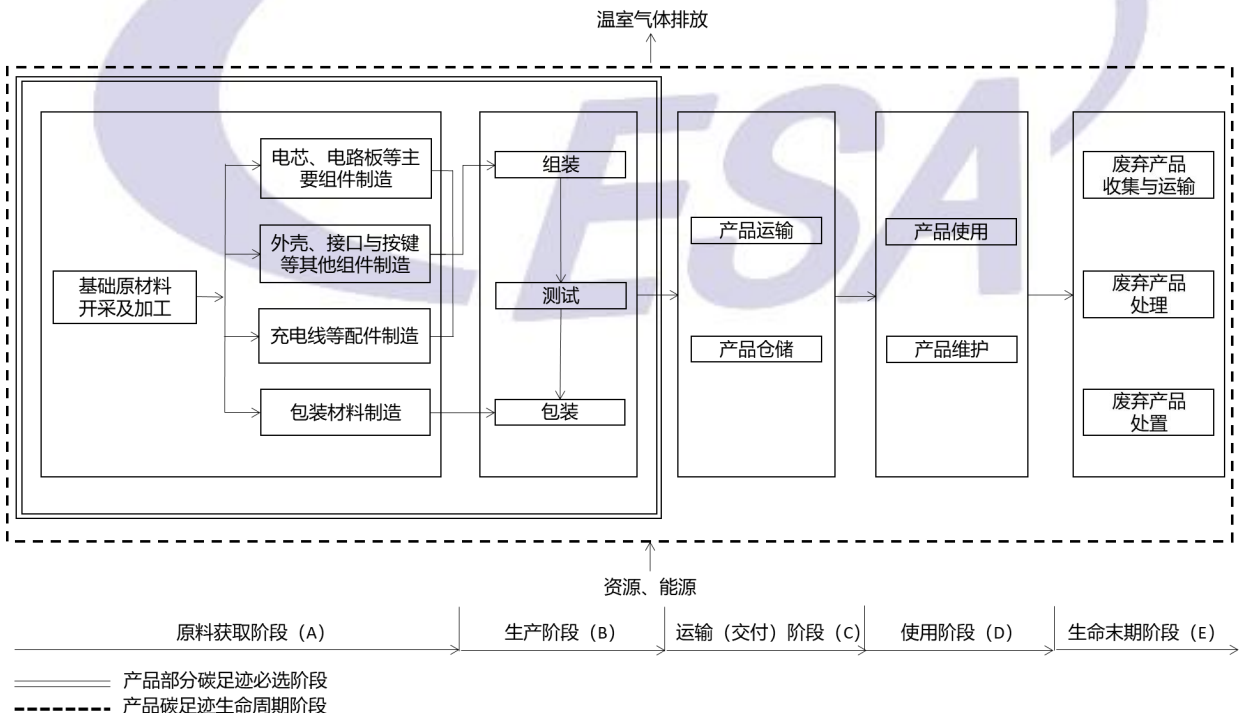
图 1 便携式移动电源产品碳足迹量化系统边界
