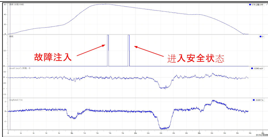
图2 功能安全试验结果示例
