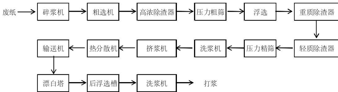
7 脱墨浆生产工艺流程图
