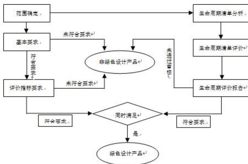
图1 卫生用品用胶粘剂绿色设计产品评价流程
