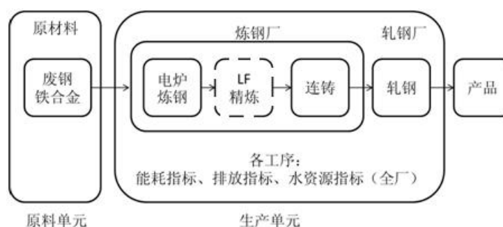
图 B.2 非调质冷镢钢用热轧盘条生命周期系统边界示意图（短流程）
