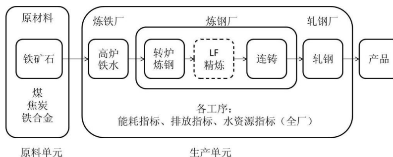
图 B.1 非调质冷镢钢用热轧盘条生命周期系统边界示意图（长流程）
