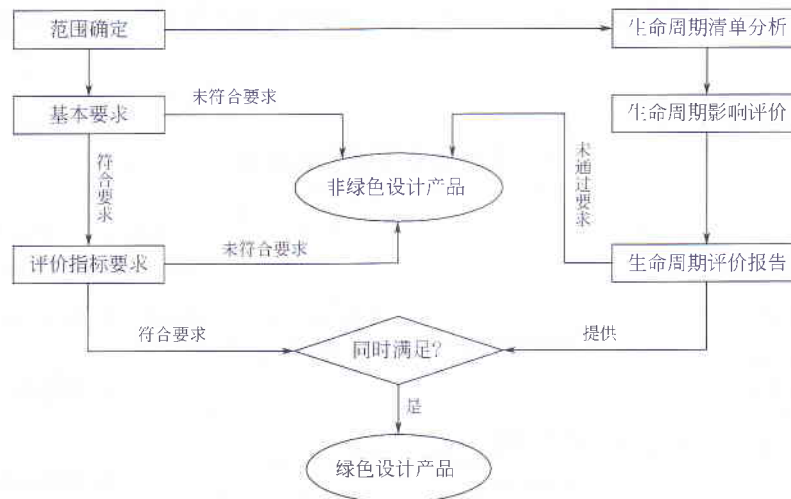
图1 碳酸钠（纯碱）绿色设计产品评价流程
