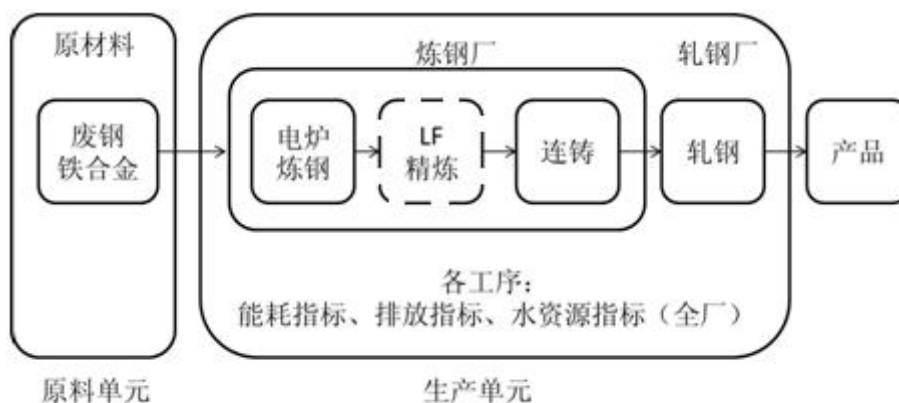
图 B.2 锚杆用热轧带肋钢筋生命周期系统边界示意图（短流程）
