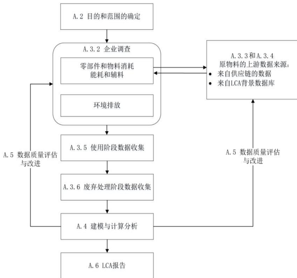
图 A.1 电吹风产品生命周期评价基本步骤
