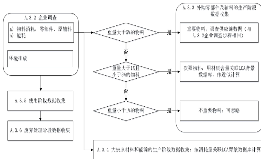
图 A.3 电吹风产品生命周期清单数据收集基本步骤
