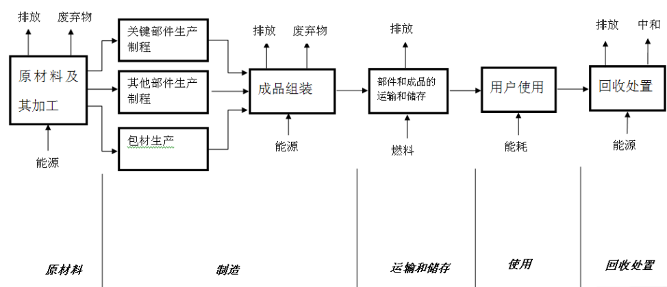
图 A.1 电动洗衣机生命周期系统边界图
