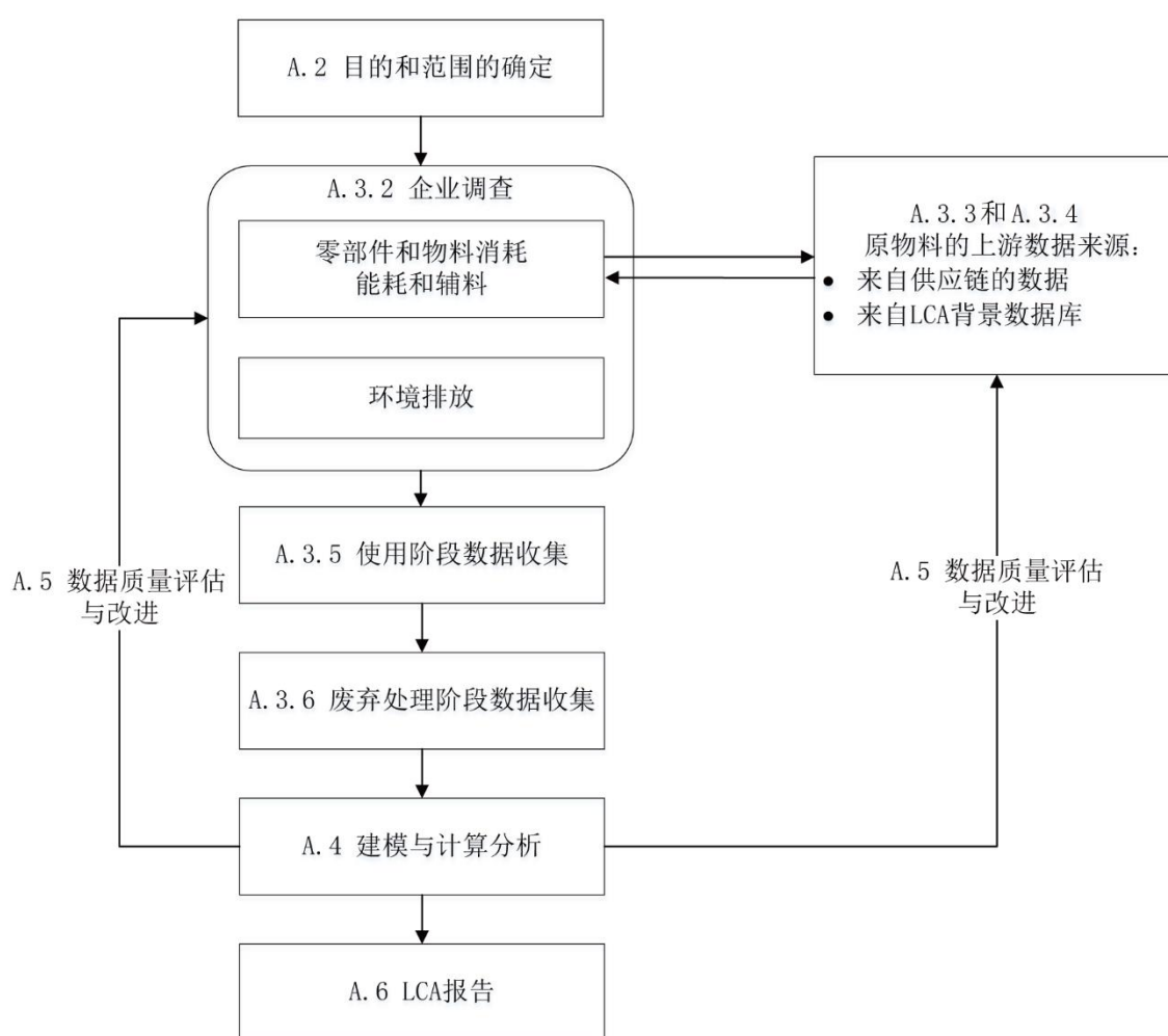
图A.1 电子电气品生命周期评价基本步骤
