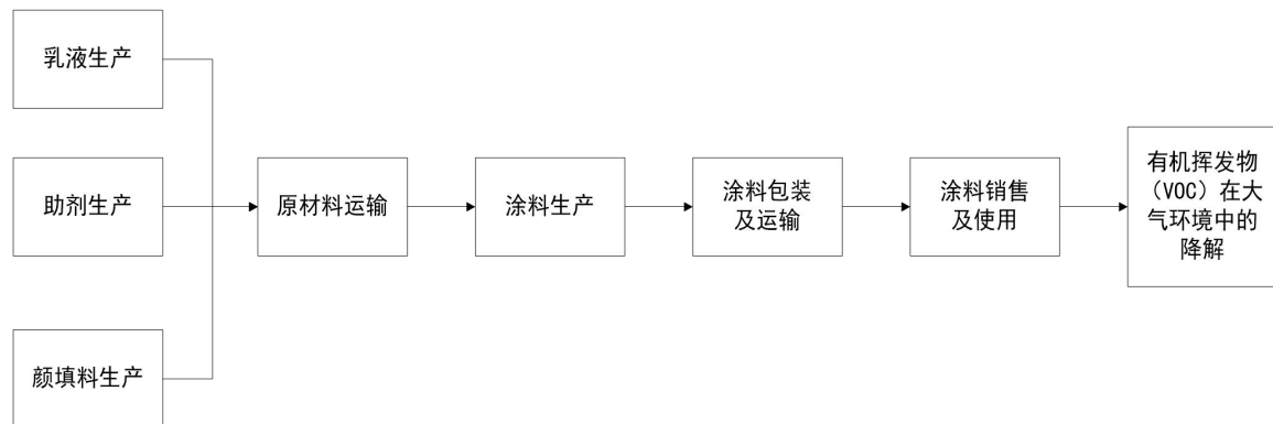
图 B.1 水性木器涂料产品生命周期（LCA）系统边界图
