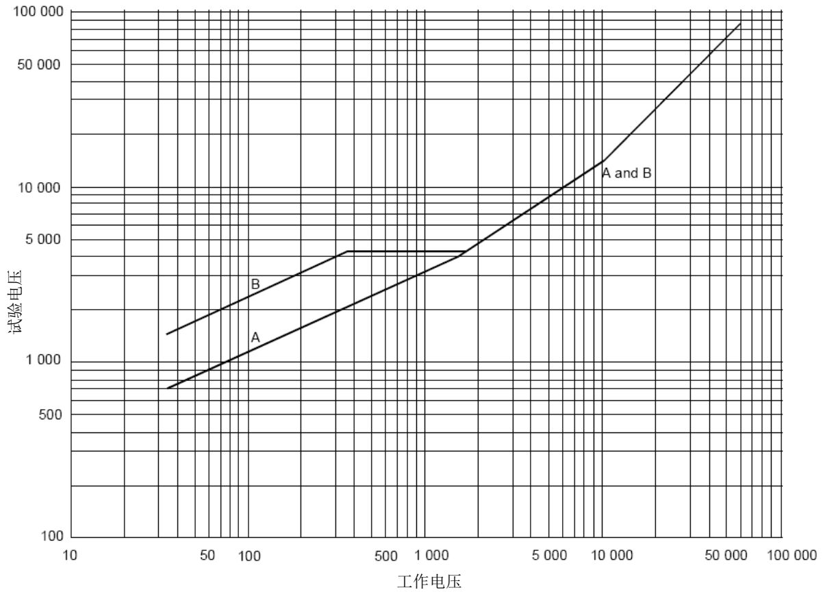
图 7 试验电压
