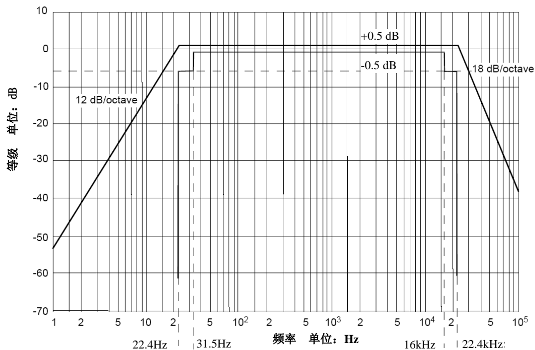
图 C.1 宽带噪声测量用带通滤波器 (幅度/频率响应限值)
