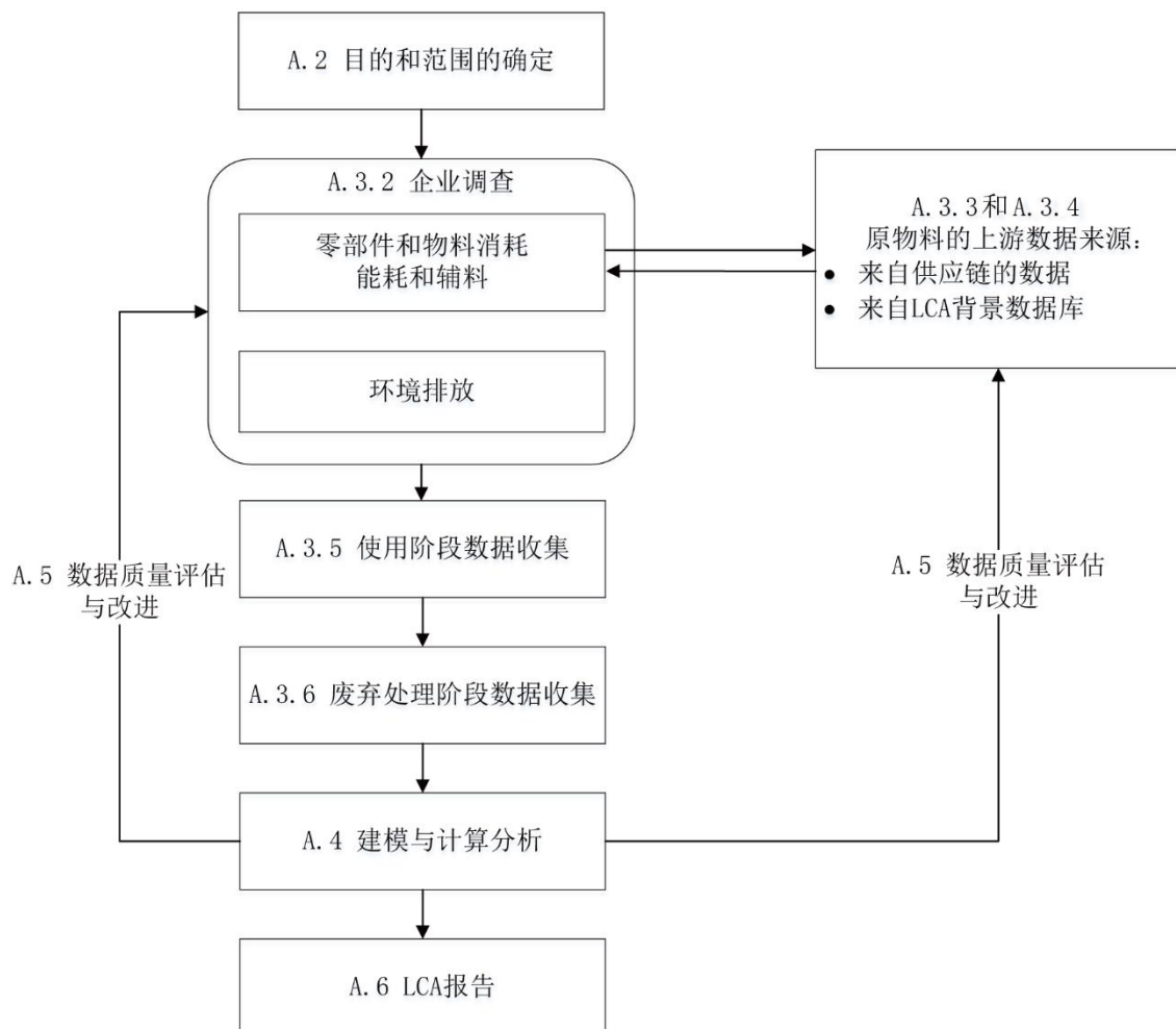
图A.1 电子电气品生命周期评价基本步骤
