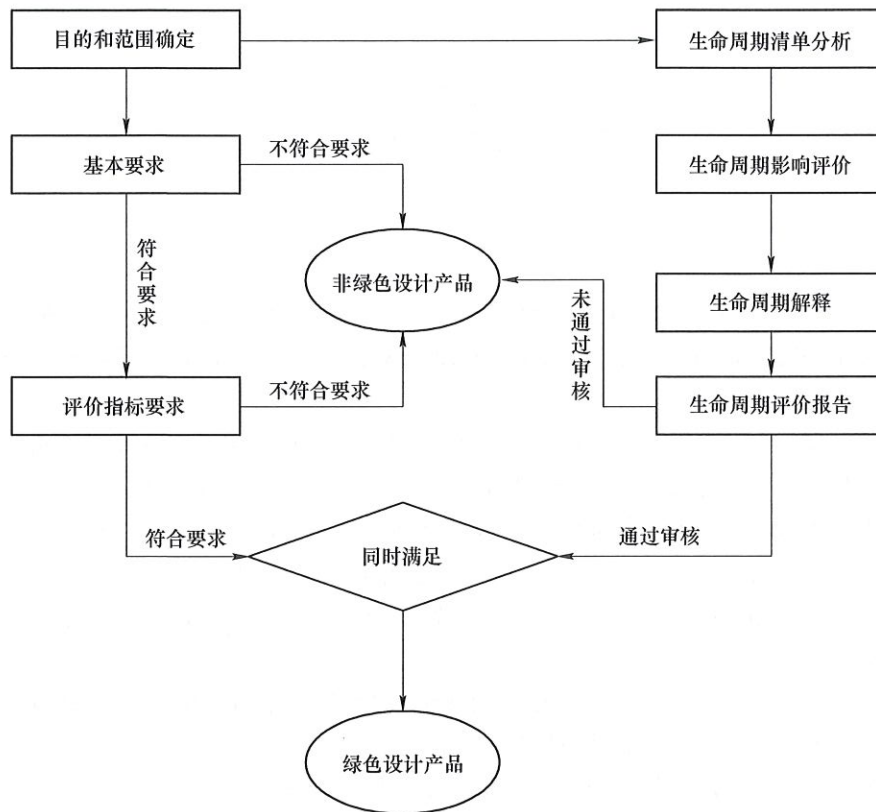
图 1 阴极铜绿色设计产品评价流程
