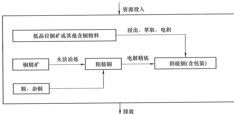
图 A.1 阴极铜产品生命周期评价的系统边界
