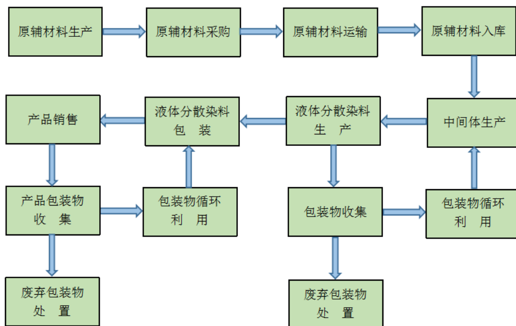
图 B.1 分散染料产品生命周期系统边界图
