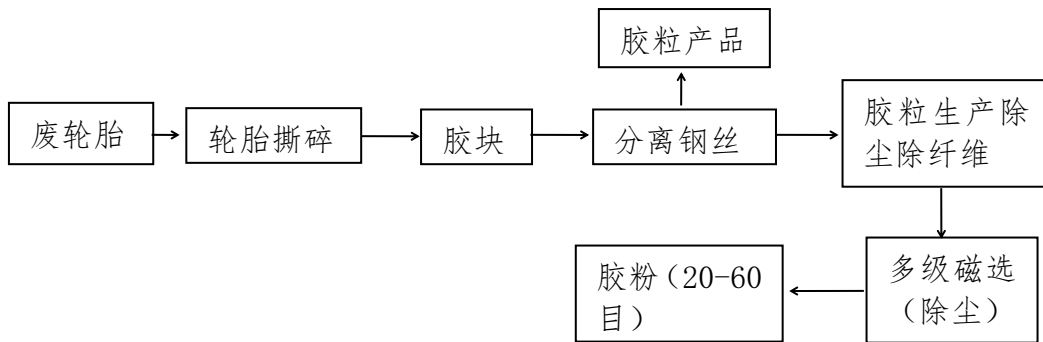
图52 环保节能型万吨级废轮胎再生橡胶技术与装备工艺流程示意图
