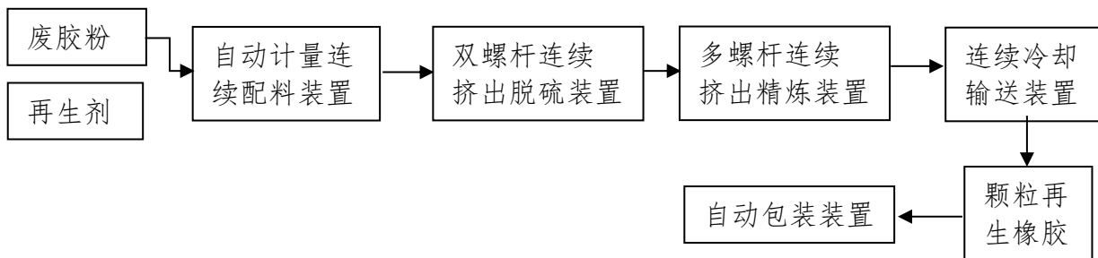
图51 多阶螺杆连续脱硫制备颗粒再生橡胶技术与装备工艺流程示意图
