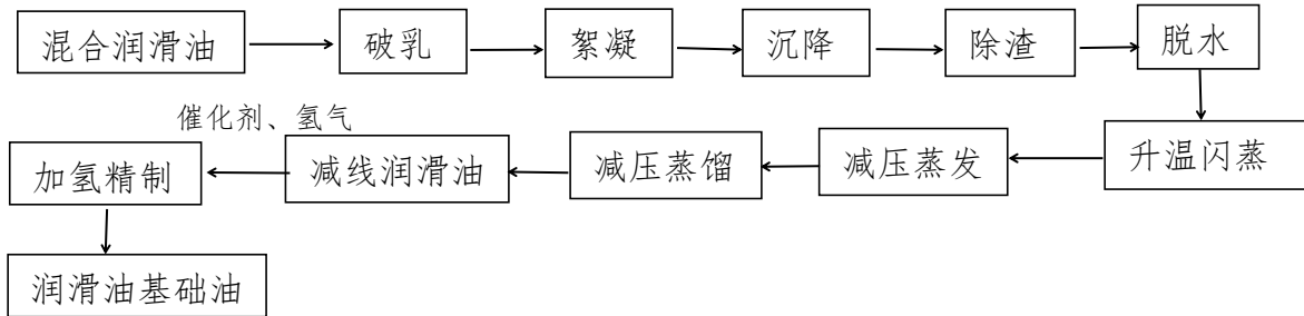
图57 废矿物油预处理加氢再生技术工艺流程示意图
