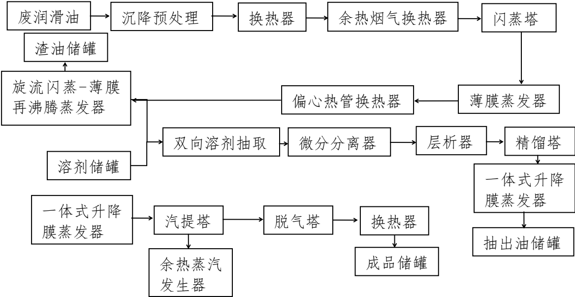
图60 旋风闪蒸-薄膜再沸+NMP双向溶剂精制技术工艺流程示意图
