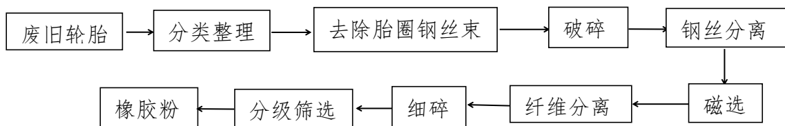
图55 废旧轮胎常温机械法制取橡胶粉技术工艺流程示意图
