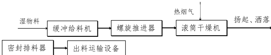
图2 滚筒干燥系统工艺流程示意图
