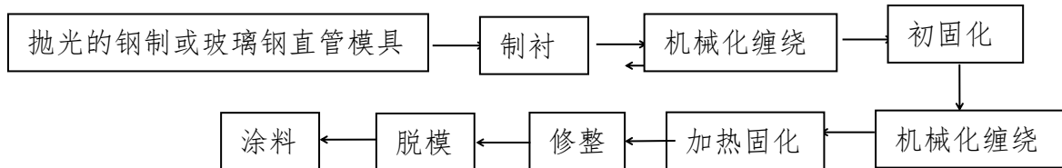
图68 竹缠绕复合管技术工艺流程示意图
