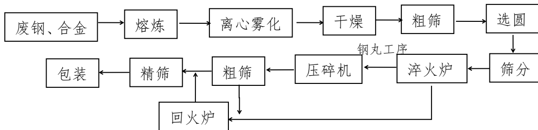
图37 HQ高碳铸钢丸生产技术工艺流程示意图
