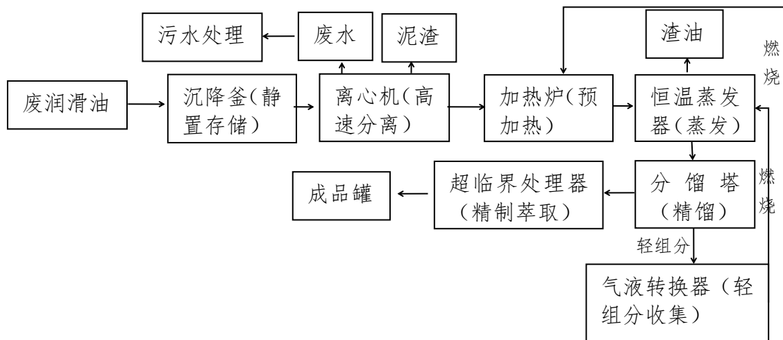
图59 废润滑油生产再生油成套装备工艺流程示意图
