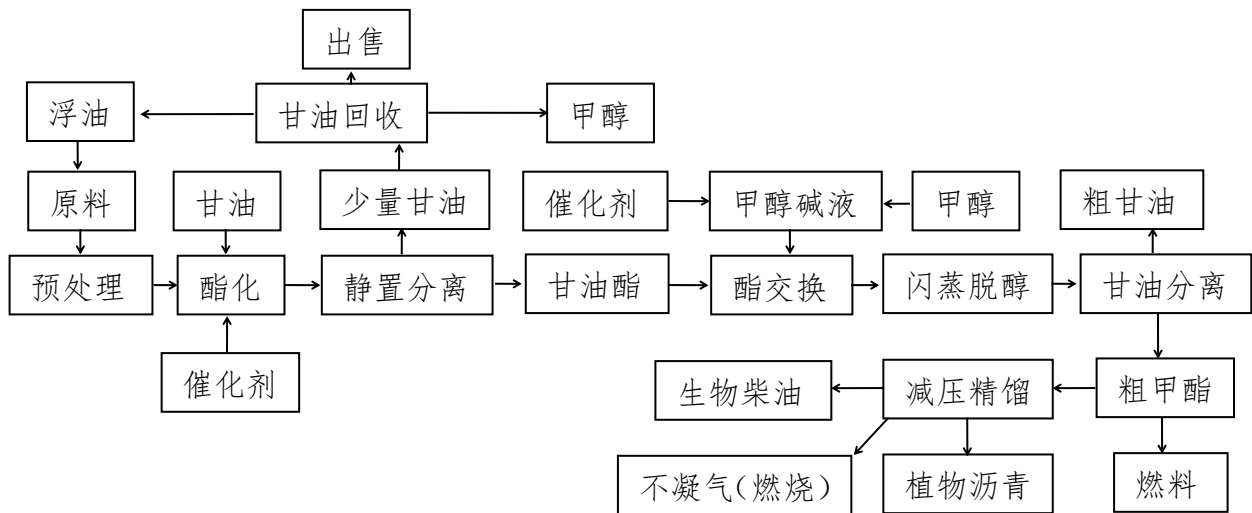
图61 生物柴油甘油酯化技术工艺流程示意图
