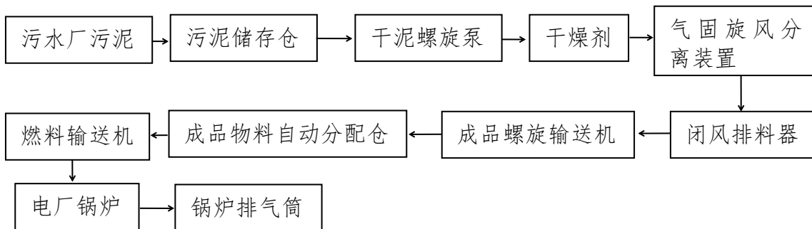
图71 市政污泥无返料干化处置技术与装备工艺流程示意图
