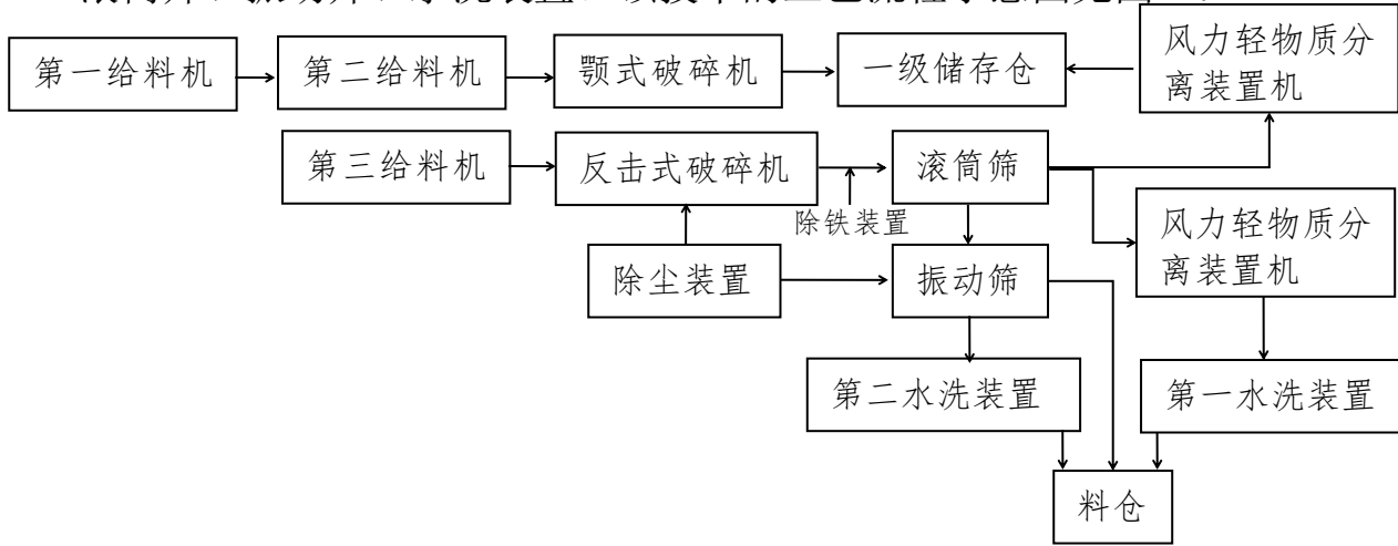
图23 建筑废弃物再生惰/活性砂粉技术工艺流程示意图
