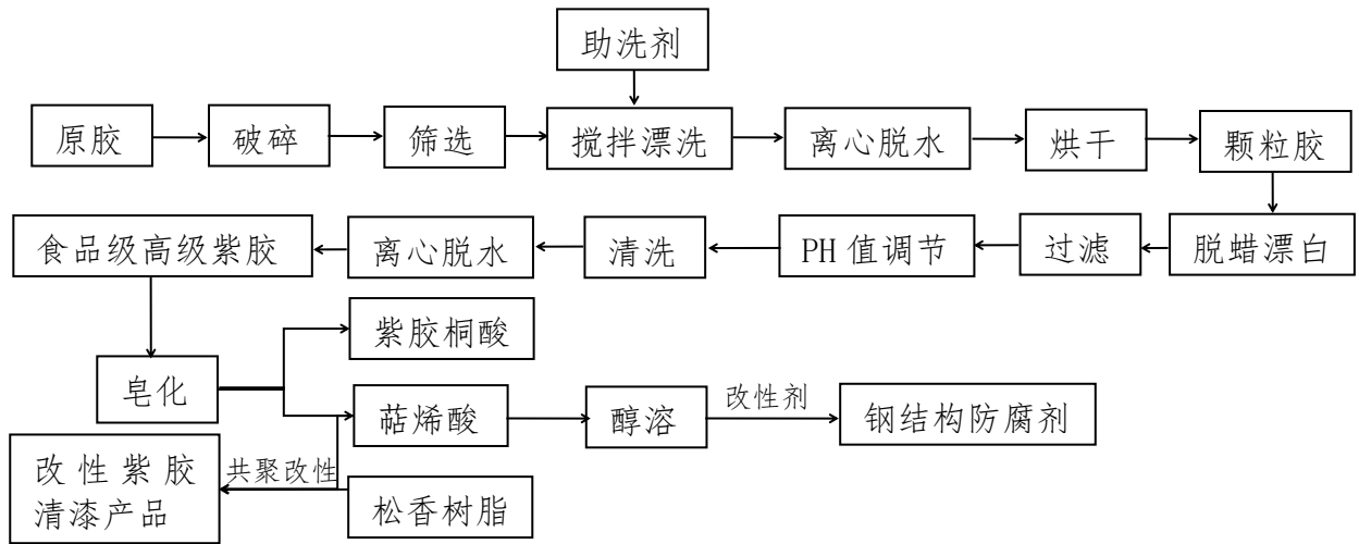
图63 紫胶桐酸提取废弃物生产钢结构防腐剂技术工艺流程示意图
