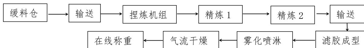
图56（3） 废橡胶智能化再生利用装备提炼成型单元工艺流程示意图
