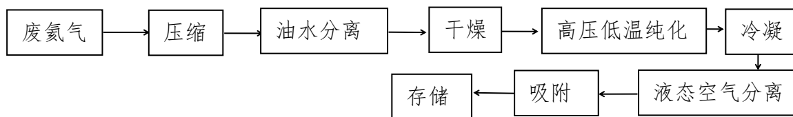
图67 工业废氨气回收利用技术与装备工艺流程示意图
