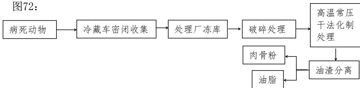
图72 病死动物高温常压无害化处理及油脂提取技术与装备工艺流程示意图
