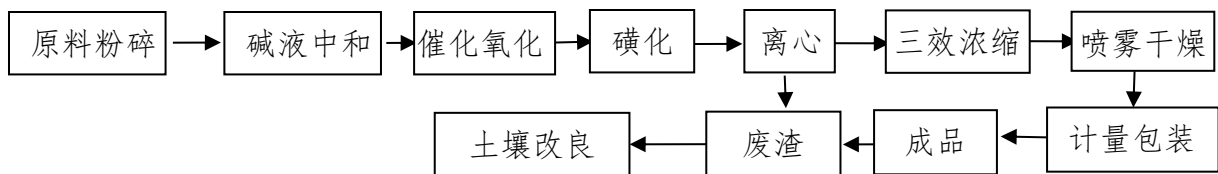
图70 风化煤催化氧化改性生产水溶性肥料专用黄腐酸钾工艺流程示意图
