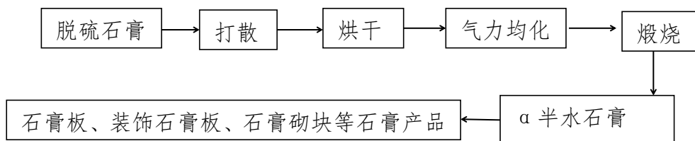
图12 工业副产石膏生产建筑石膏和纸面石膏板装备技术 工艺流程示意图
