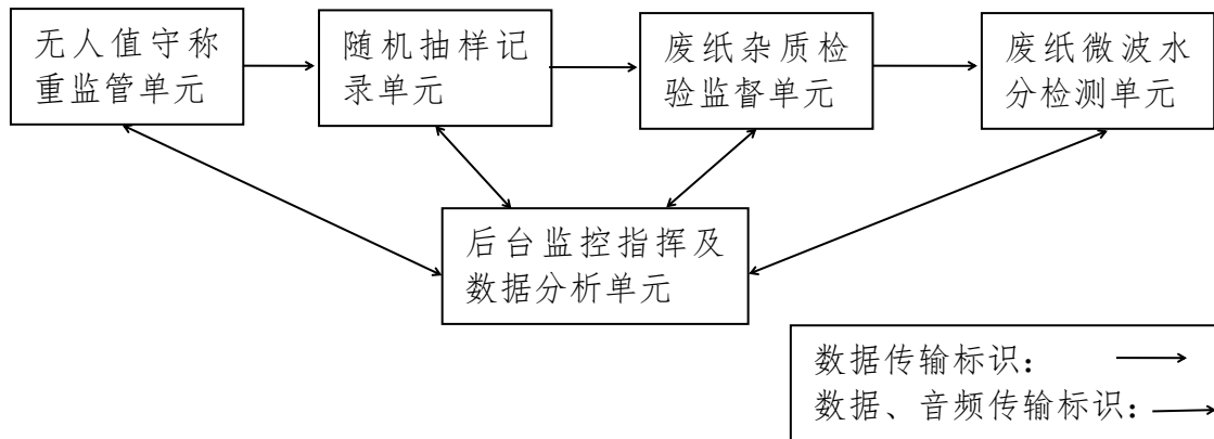
图66 基于物联网的废纸验收管理系统工艺流程示意图
