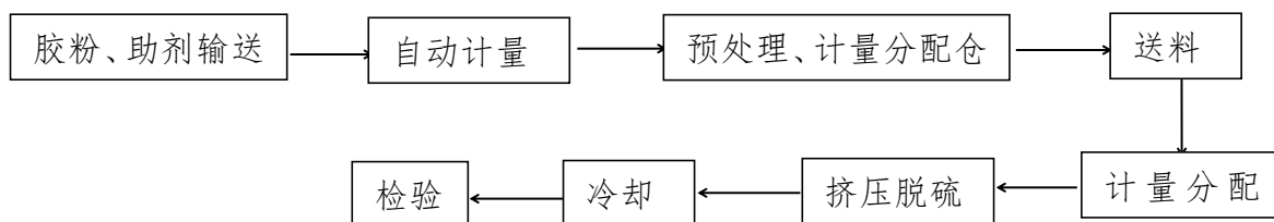
图56（2） 废橡胶智能化再生利用装备塑化单元工艺流程示意图
