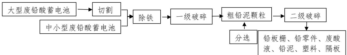
图44 废铅酸蓄电池全自动破碎分选技术工艺流程示意图
