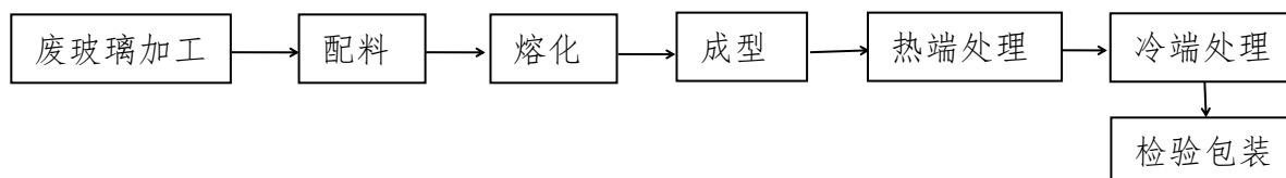
图64（2） 废玻璃分拣处理后再生产啤酒瓶技术与装备啤酒瓶制作工艺流程图示意图
