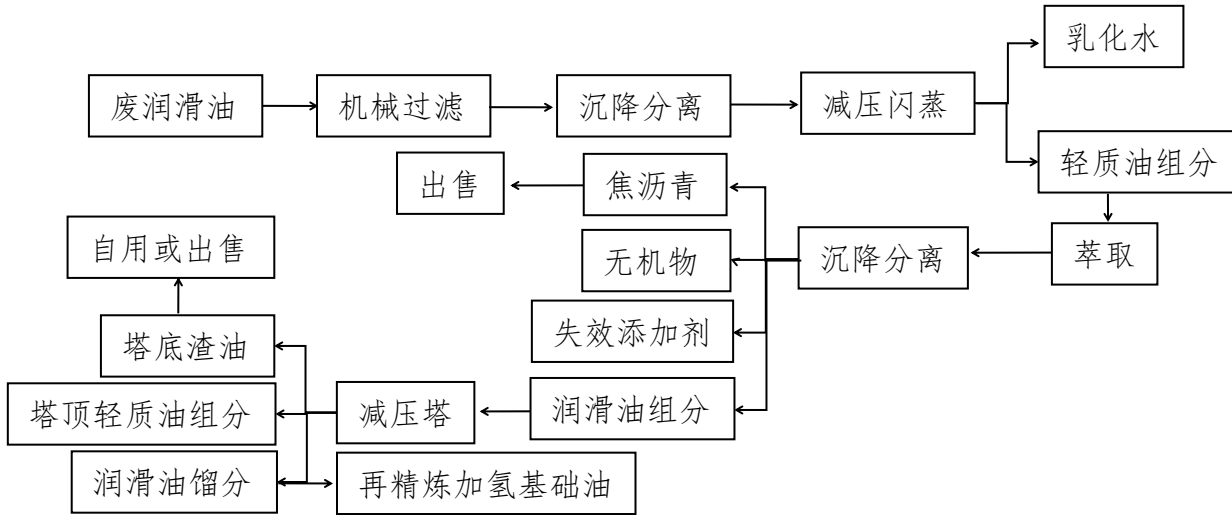
图58 废润滑油再精炼技术工艺流程示意图
