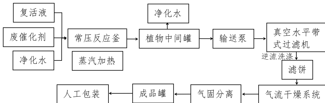
图65 FCC废催化剂复活技术与装备工艺流程示意图
