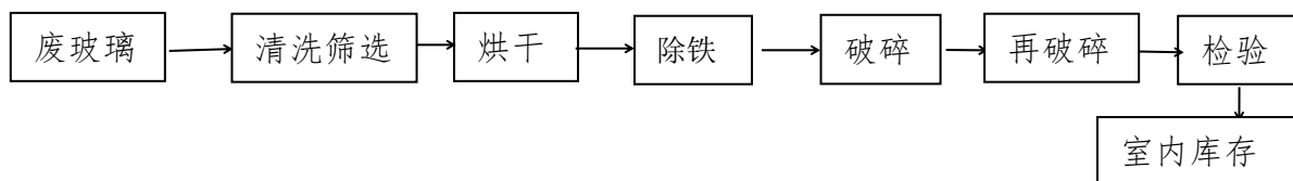
图64（1） 废玻璃分拣处理后再生产啤酒瓶技术与装备清洗破碎工艺流程示意图
