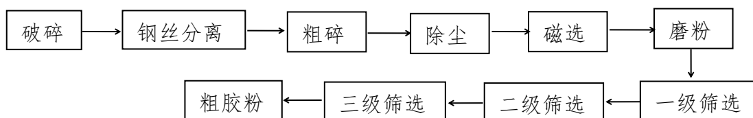
图56 废轮胎常温双轴全封闭自动化破碎技术工艺流程示意图
