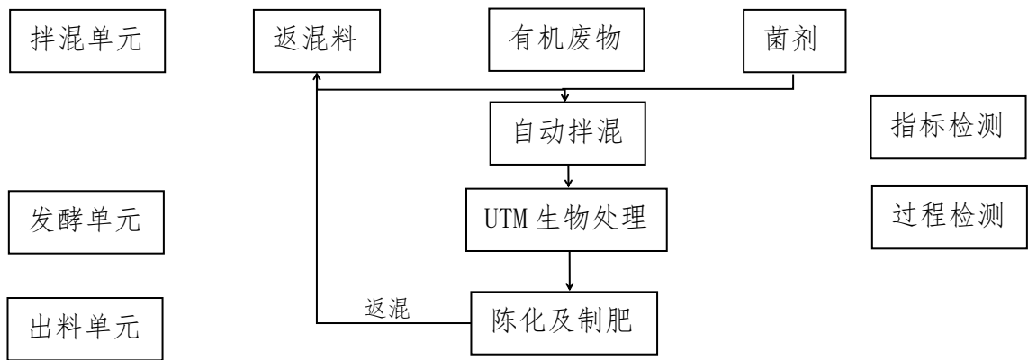
图69 有机固体废物UTM超高温好氧生物处理技术工艺流程示意图
