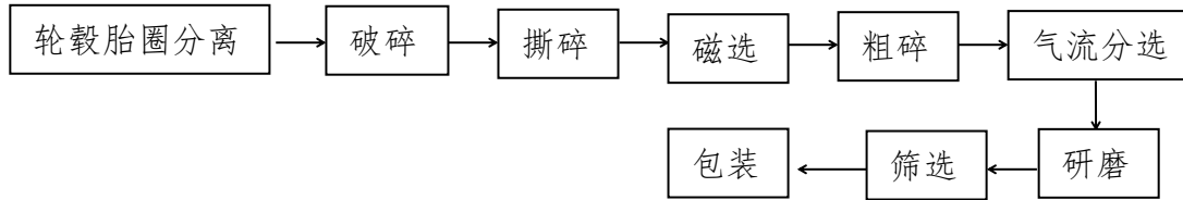
图54 节能型废轮胎自动化粉碎技术与装备工艺流程示意图
