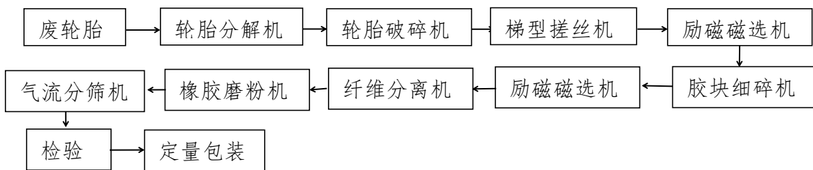
图56（1）废橡胶智能化再生利用装备粉碎单元工艺流程示意图
