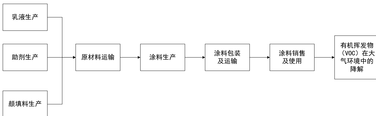
图 B.1 水性木器涂料产品生命周期（LCA）系统边界图
