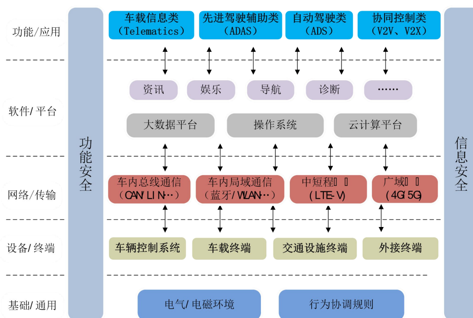
图 2 智能网联汽车产品物理结构
